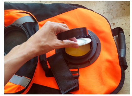
3. Extraer el anillo interior y el filtro de la mochila.
